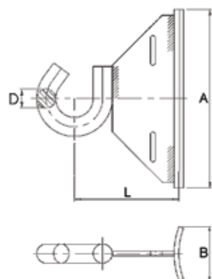
HEL-553x
