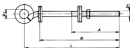
HEL-555x
